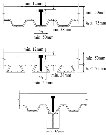
Şekil 12.4 – Şekil verilmiş çelik sac için konstrüktif esaslar
