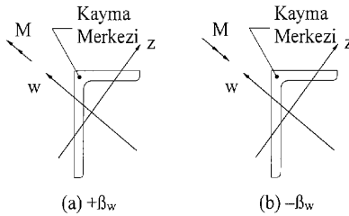
Şekil 9.2 – Eğilme momenti etkisindeki farklı kollu korniyerler için \beta_w işareti tanımı
