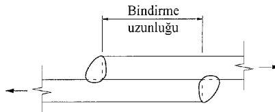
Şekil 13.5 – Minimum bindirme uzunluğu
