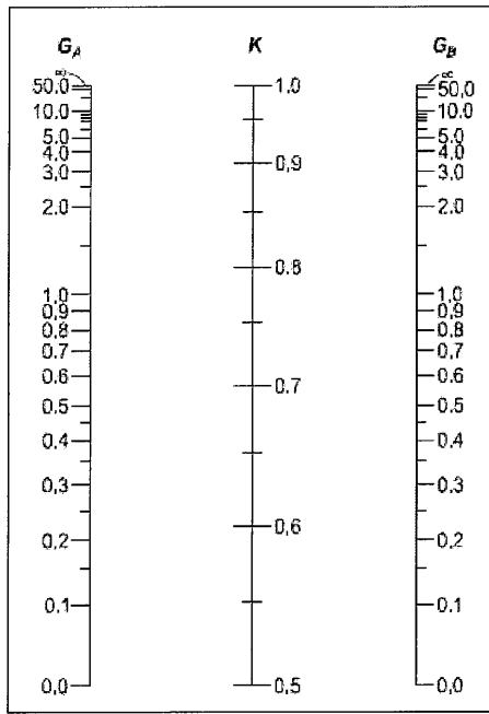
Şekil 6.1 – Yanal yerdeğiřtirmesi önlenmiř sistemlerde burkulma boyu katsayısı, K
