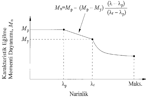
Şekil 12.5- Beton dolgulu kompozit kirişlerde karakteristik eğilme momenti dayanımı
