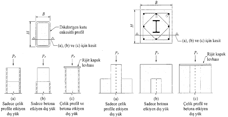
Şekil 12.8 – Kompozit kolonda dış yük etkisi
