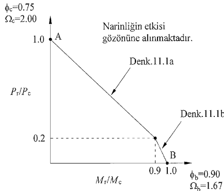
Şekil 12.6 – Kompozit elemanlar için genel etkileşim diyagramı
