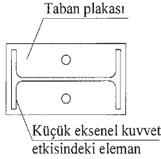
Şekil 13.10 – Küçük eksenel kuvvet etkisindeki elemanların ankrajı
