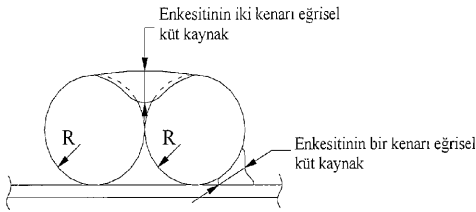
Şekil 13.2 – Enkesiti eğrisel kenarlı küt kaynaklar
