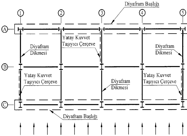
Şekil Ek 3.1 – Tipik yük aktarma elemanları (diyafram dikkeleri) ve diyafram başlıkları
