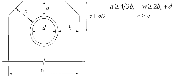
Şekil 13.11 – Çekme elemanlarının mil birleşimleri için boyutlar
