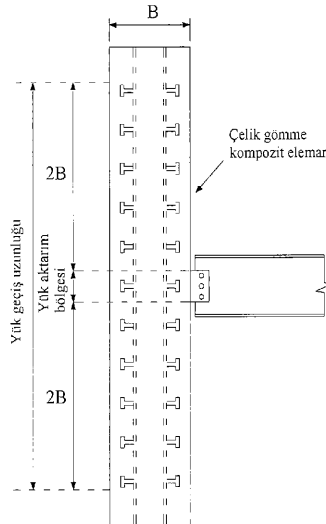
Şekil 12.9 – Yük aktarım bölgesi ve yük geçiş uzunluğu
