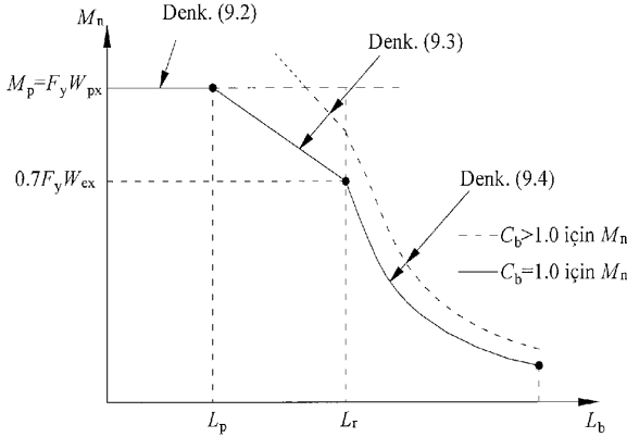
Şekil 9.1 – Basınç başlığının yanal olarak desteklenmeyen uzunluğuna bağlı olarak karakteristik eğilme momenti dayanımı
