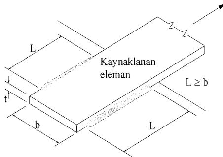
Şekil 13.3 – Sadece boyuna kaynak uygulanan uç birleşimi
