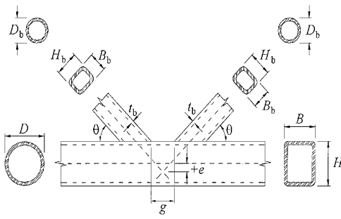
(a) Ara uzaklıklı K-birleşimi
