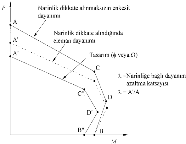
Şekil 12.7 – Kompozit elemanlar için geliştirilmiş karşılıklı etki diyagramı
