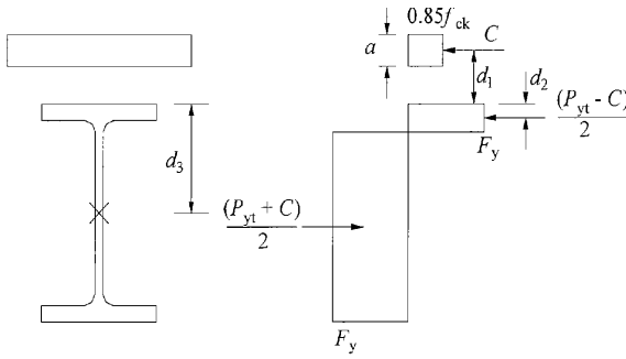
Şekil 12.2 – Kompozit kirişte pozitif eğilme momenti için genel plastik gerilme yayılımı
