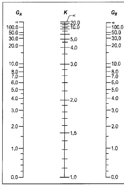
Şekil 6.2 – Yanal yerdeğiştirmesi önlenmemiş sistemlerde burkulma boyu katsayısı, K
