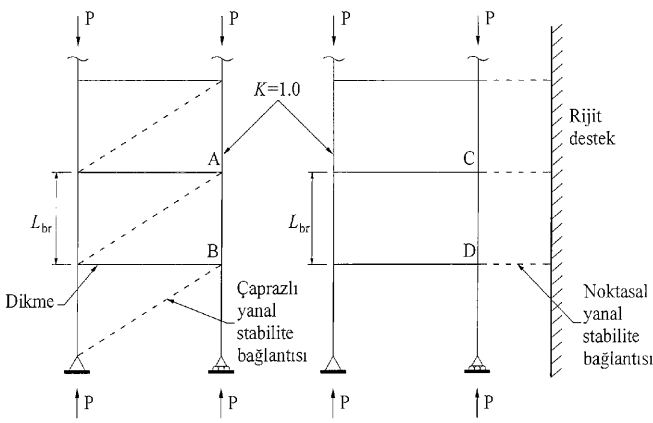
Şekil 16.1 – Kolonlar için stabilite bağlantıları
