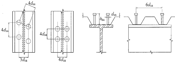
Şekil 12.11 – Başlıklı çelik ankrajların yerleşimi
