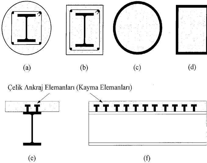
Şekil 12.1 – Tipik kompozit elemanlar
