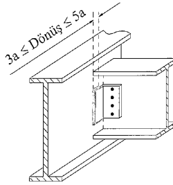
Şekil 13.7 – Kiriş ucu ile birleşim elemanı arasında dönme uyumunun sağlanabilmesi için kaynak uygulaması
