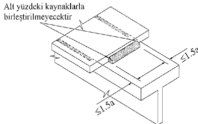
Şekil 13.8 – Bir düzlemin farklı yüzeylerindeki köşe kaynaklar için uygulama detayı
