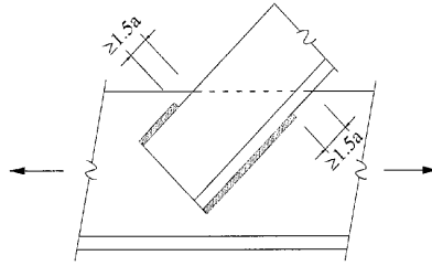
Şekil 13.6 – Çekme etkisindeki bir elemana köşe kaynaklı bağlantı
