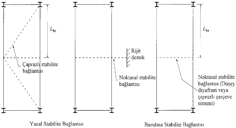
Şekil 16.2 – Kirişler için stabilite bağlantıları
