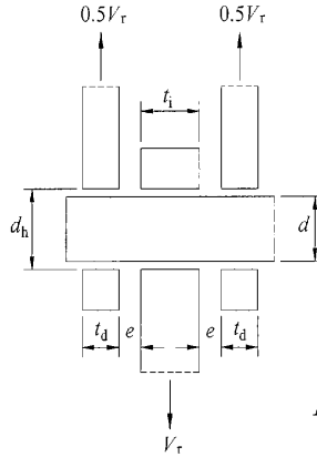
Şekil 13.12 – Çekme elemanlarının mil birleşimleri için gerekli dayanımlar
