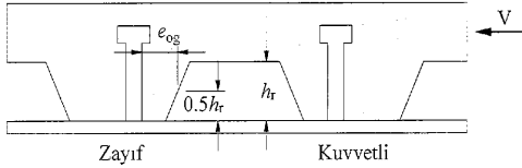
Şekil 12.10 – Ankrajların kesme kuvveti etkisinde kuvvetli ve zayıf olarak yerleşimi
