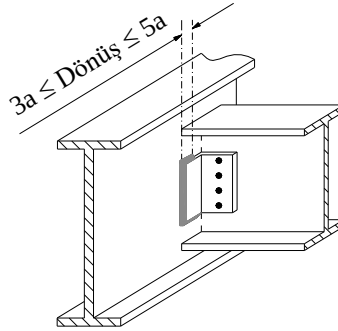
Şekil 13.7 – Kiriş ucu ile birleşim elemanı arasındaki dönme uyumunun sağlanabilmesi için kaynak uygulaması
