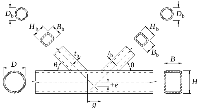
(a) Ara uzaklıklı K-birleşimi
