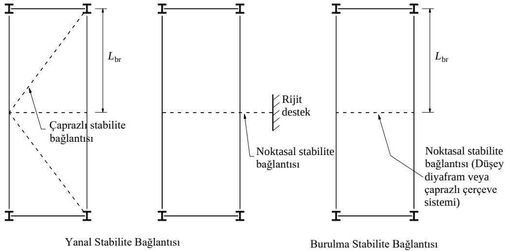
Şekil 16.2 – Kirişler için stabilite bağlantıları
