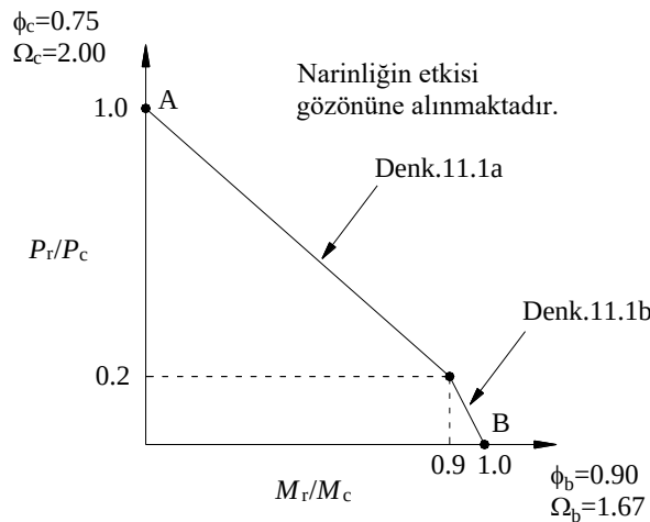
Şekil 12.6 – Kompozit elemanlar için genel etkileşim diyagramı
