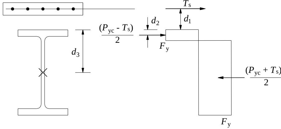
Şekil 12.3 – Kompozit kirişte negatif eğilme momenti için genel plastik gerilme yayılımı
