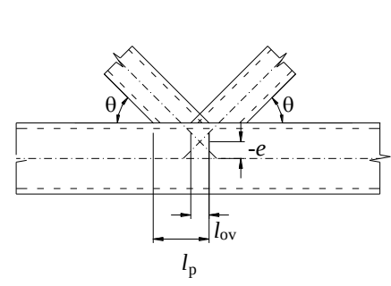
(b) Bindirmeli K-birleşimi
