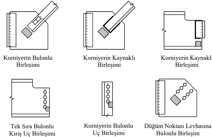
a) U_{bs} = 1.0 olan birleşim tipleri
