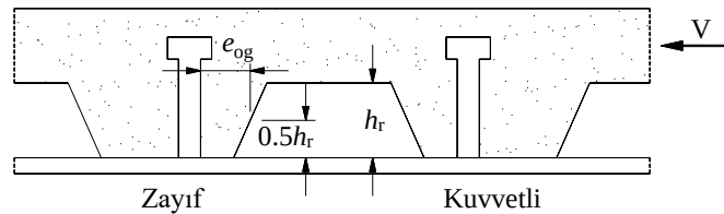
Şekil 12.10 – Ankrajların kesme kuvveti etkisinde kuvvetli ve zayıf olarak yerleşimi
